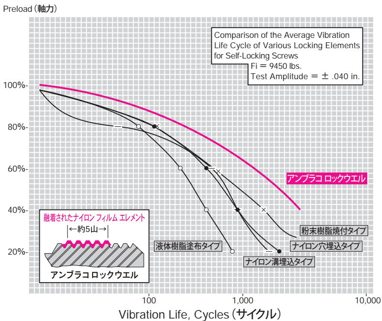
■ SPS振動試験機による軸力損失比較データ (米国SPS Laboratories)
